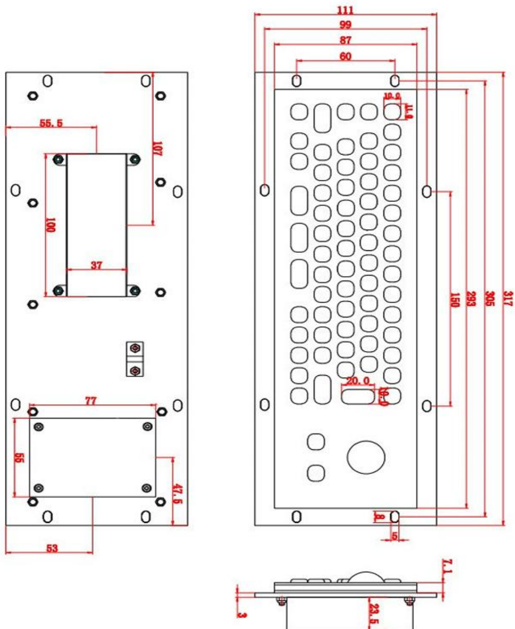
Rysunek techniczny klawiatury RuggedKEY model RMKB705-BL
