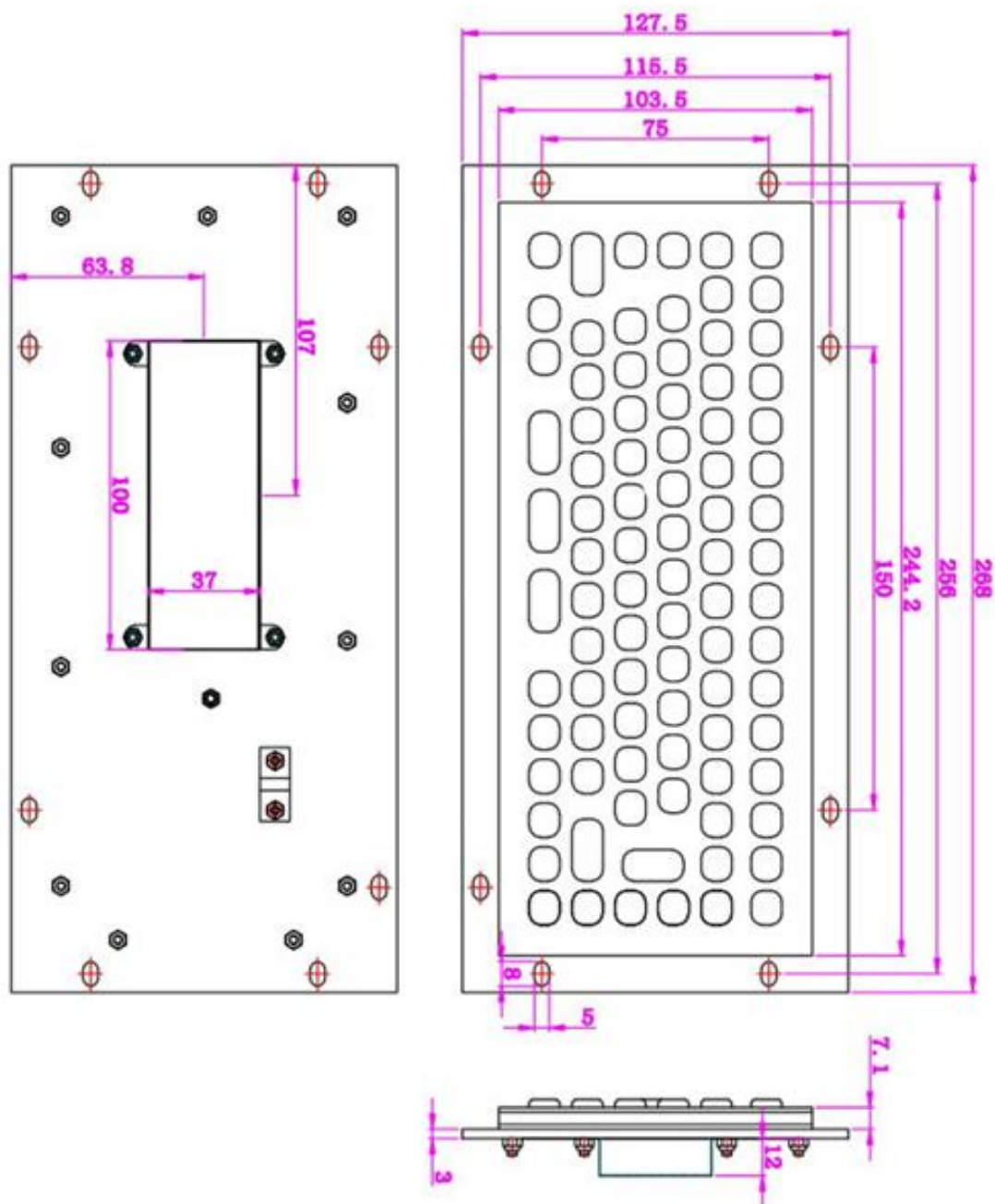
Rysunek techniczny klawiatury RuggedKEY model RMKB702
